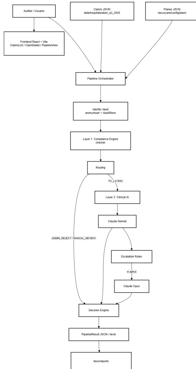
FIGURA VII.1 : Workflow del sistema: flujo de cinco fases desde la liquidación hasta la decisión del auditor.
