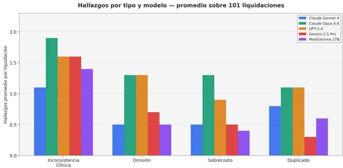
FIGURA X.2: Promedio de hallazgos por liquidación, por tipo y modelo.
