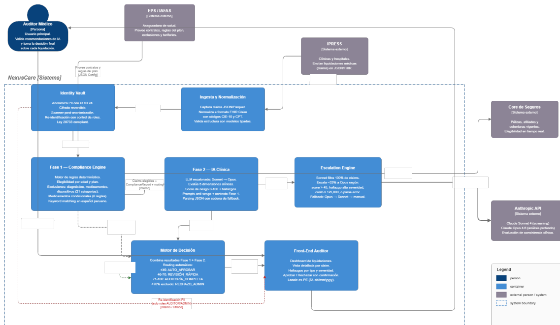
FIGURA VII.3: Diagrama C4 de contenedores del sistema.
